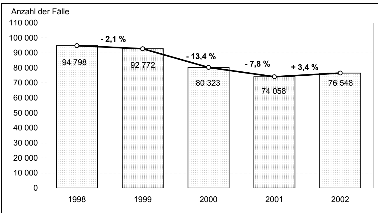
Abbildung 41: Entwicklung der Straßenkriminalität
