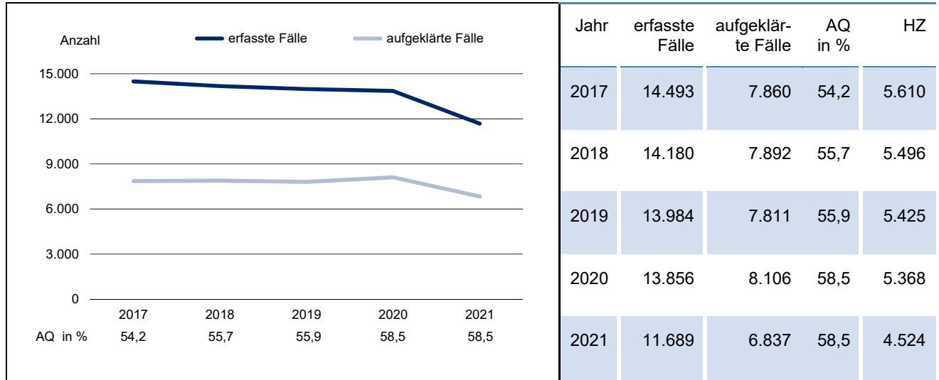
erfasste Fälle 2017 - 2021
