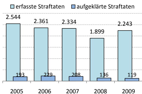
Abbildung 8: Entwicklung Fahrraddiebstähle
