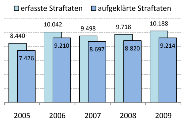
Abbildung 9: Entwicklung Betrug
