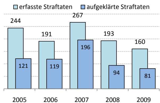
Abbildung 7: Entwicklung Brandstiftung
